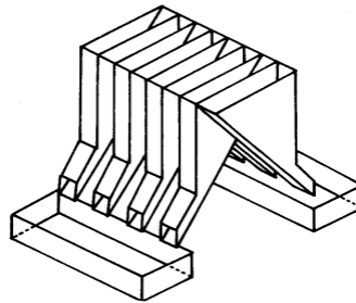
Fig. 22. Box divider.
